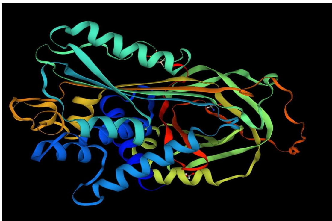
Figura 2: Modelagem tridimensional da proteína fXa em que cada cor representa uma sequência terciária ou quaternária de aminoácidos, formando folhas alfa, cores laranja, amarelo e vermelha e folhas beta, cores azuis (todos os tons) e verde (todos os tons)
